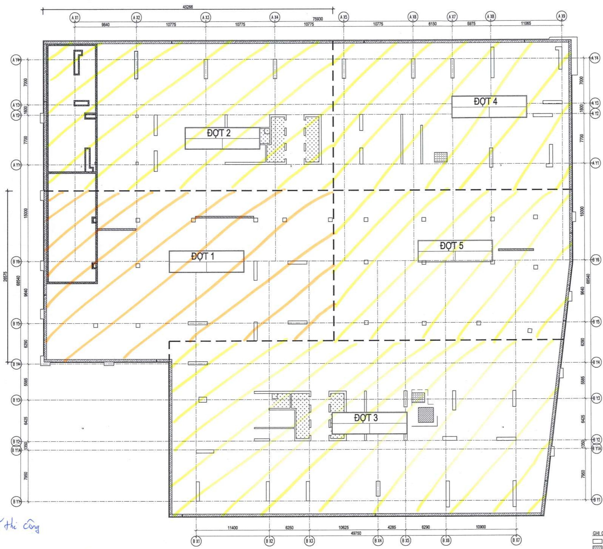
MẶT BẰNG KẾ HOẠCH THI CÔNG SÀN HẦM B1 THÁNG 9/2024
